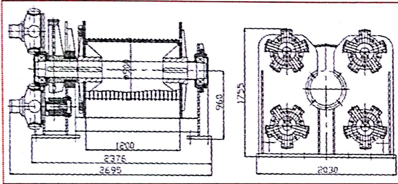
YHJ350 液压绞车 Hydraulic Winch
