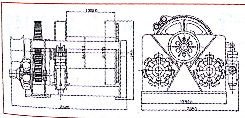
YB180液压绞车 Hydraulic Winch
