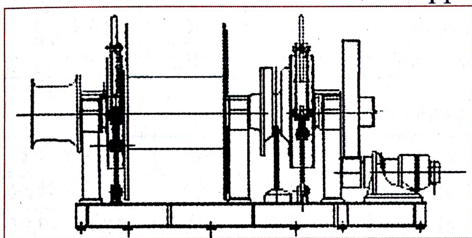
液压绞车 Hydraulic Winch
