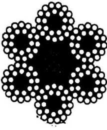
6×24+7FC
