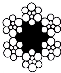
6×9W+FC
