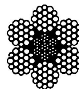
6 × 19W+IWR
