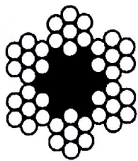
6×7+FC
