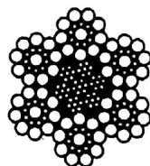
6 × 19S+IWR
