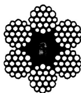
6 × 19W+FC
